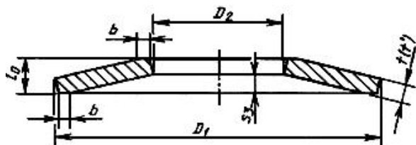
Пружина типа 2
