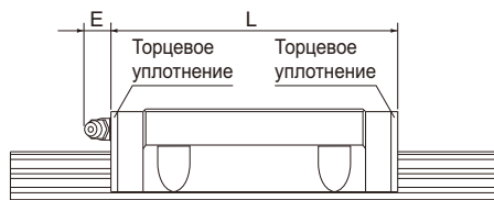
Рис.1 Размеры смазочного ниппеля для модели SHW
