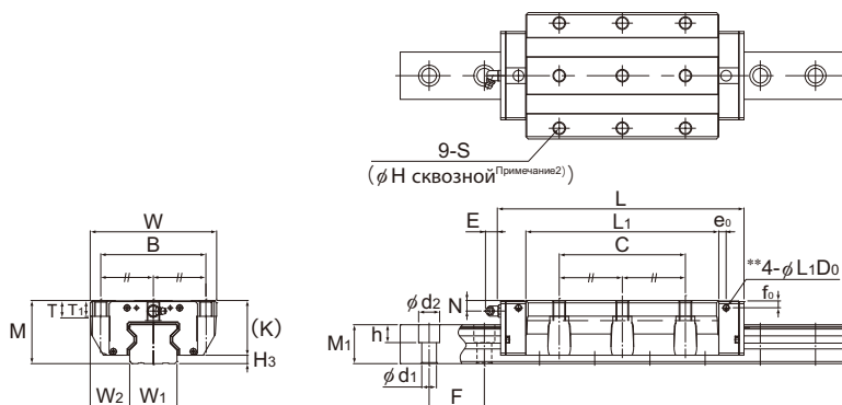
Модели SRG35 до 65 SLC
