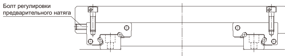
Рис.1 Пример регулировки предварительного натяга с помощью нажимного болта
