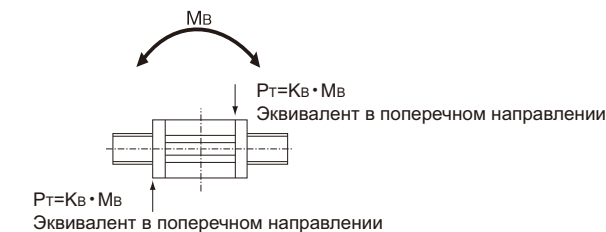
Рис.4 Коэффициенты приведенного момента M_B
