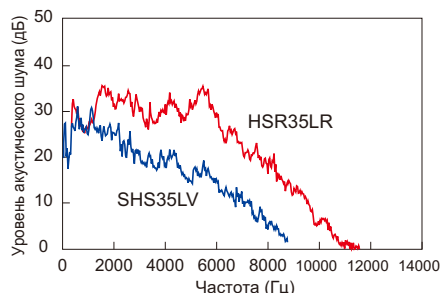
Сравнение уровня шума у моделей SHS35LV и HSR35LR (при скорости 50 м/мин)
