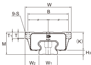
Модели HSR100 до 150HA
