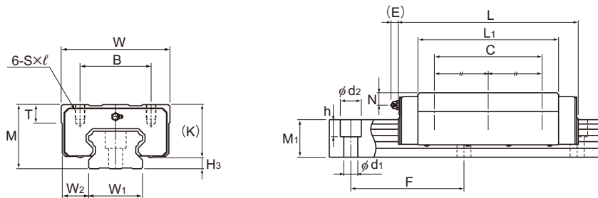
Модели HSR100 до 150HR
