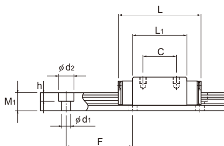
Модели HSR8RM и 10RM
