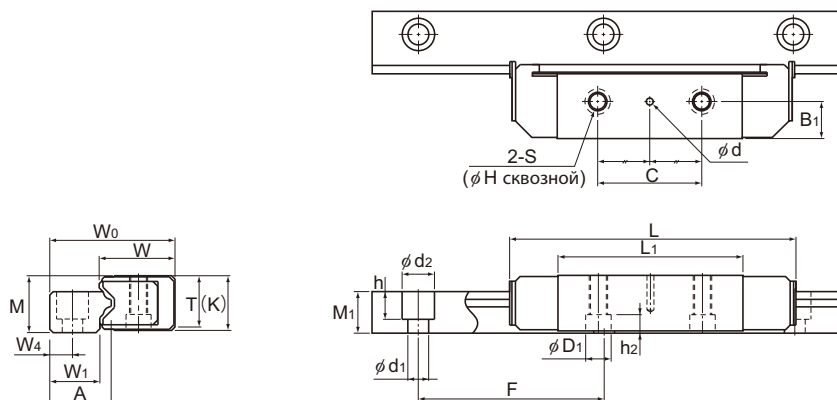
Модели HR1123 до 2555M/T/TM
