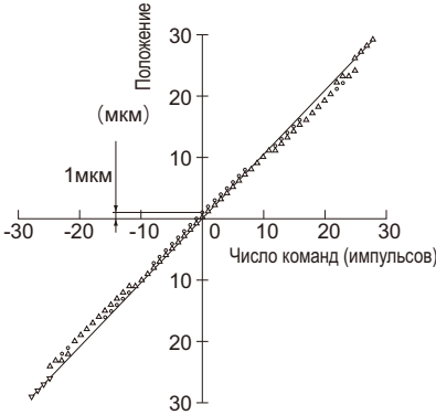
Направляющая LM модели HSR45
