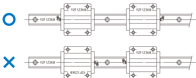
Рис.22 Маркировка серийного номера и комбинированное использование рельса и кареток LM
