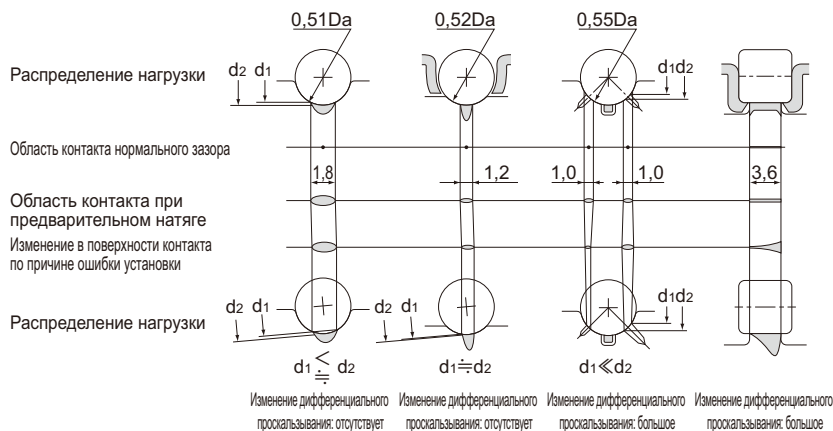
Рис.4 Сравнение контактной поверхности (φ 6,350 шарик, φ 6 x 6l ролик)
