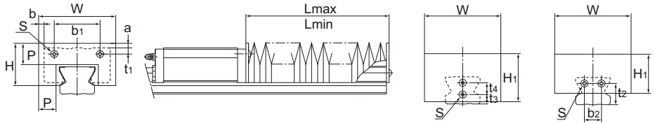
Модели с SR15 по 25 Модели с SR30 по 70 Един. измер.: мм
