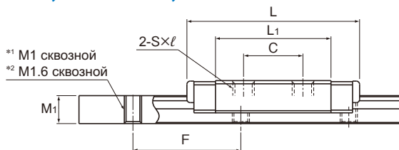
Модель RSR2N, RSR3N
