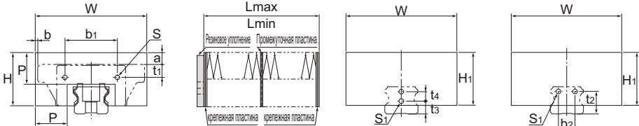
Модели с SHS15 по 30 Модели с SHS35 по 65
