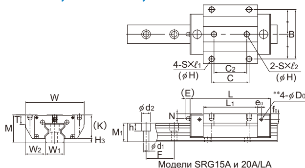
Модели SRG15A и 20A/LA
