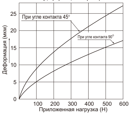
Нагрузка и деформация при разных углах контакта ( Da=6,35 мм) (деформация шарика)
