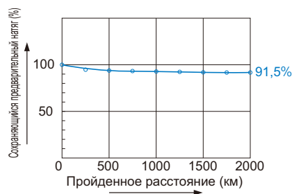
Рис.7 Пройденное расстояние и оставшийся преднатяг
