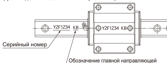
Рис.12 Основной рельс LM
