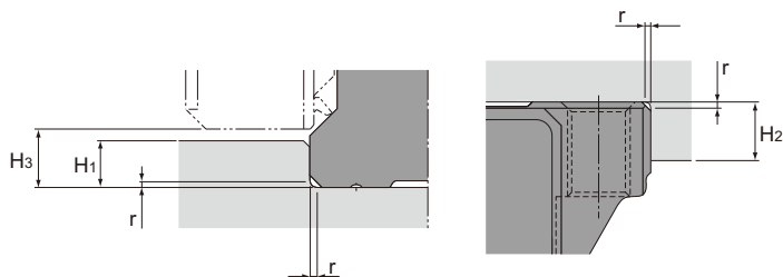
Плечо для рельса LM
